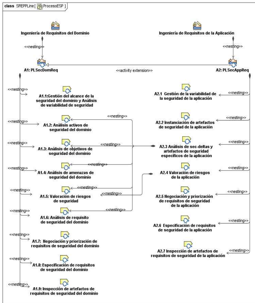
Fig. 1 Especificación de las actividades de SREPPLine usando SPDM 2.0
